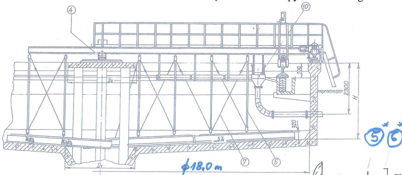
Zgarniacz osadu typu ZURc (przekrój pionowy)
